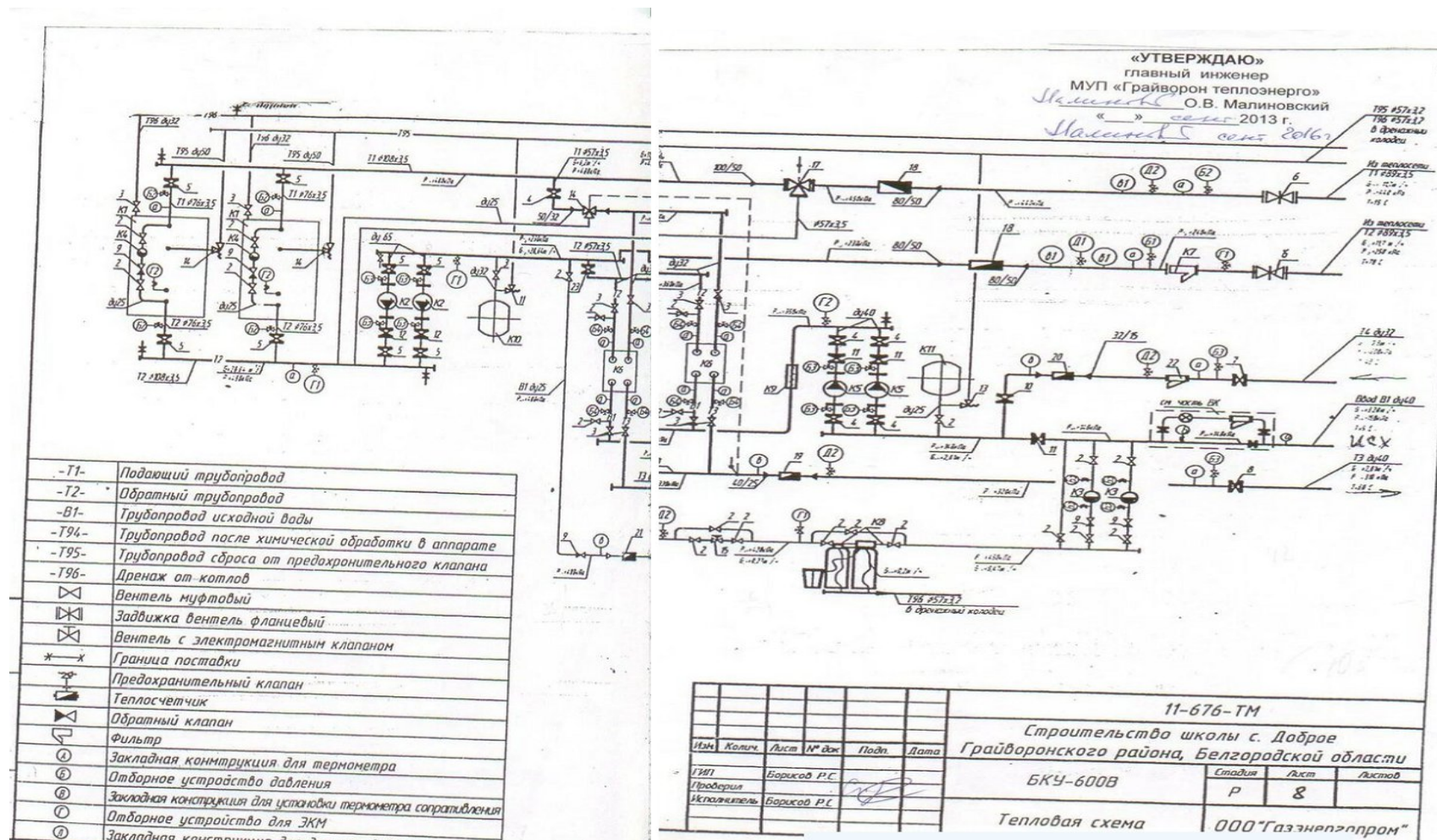
Рисунок 24. Тепловая схема котельной Доброе
