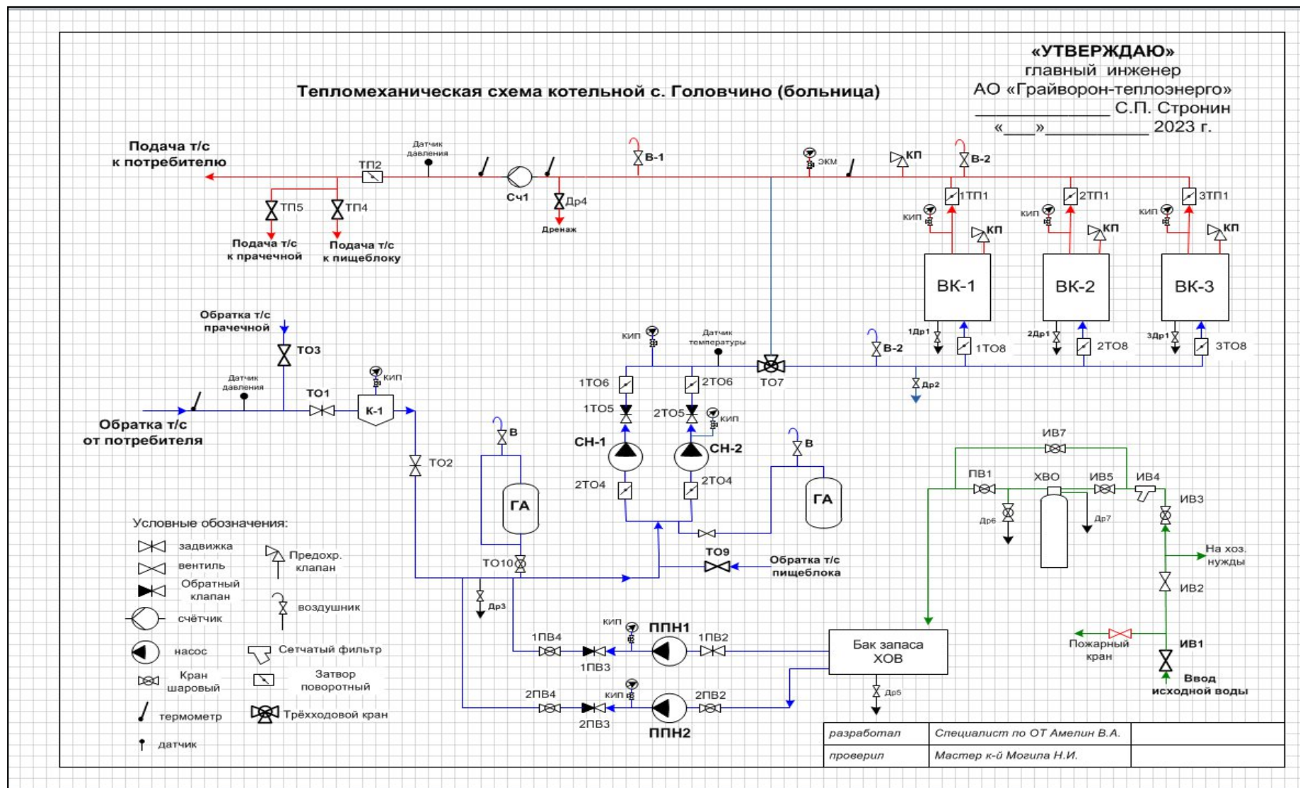
Рисунок 28. Тепловая схема котельной с. Головчино (больница)
