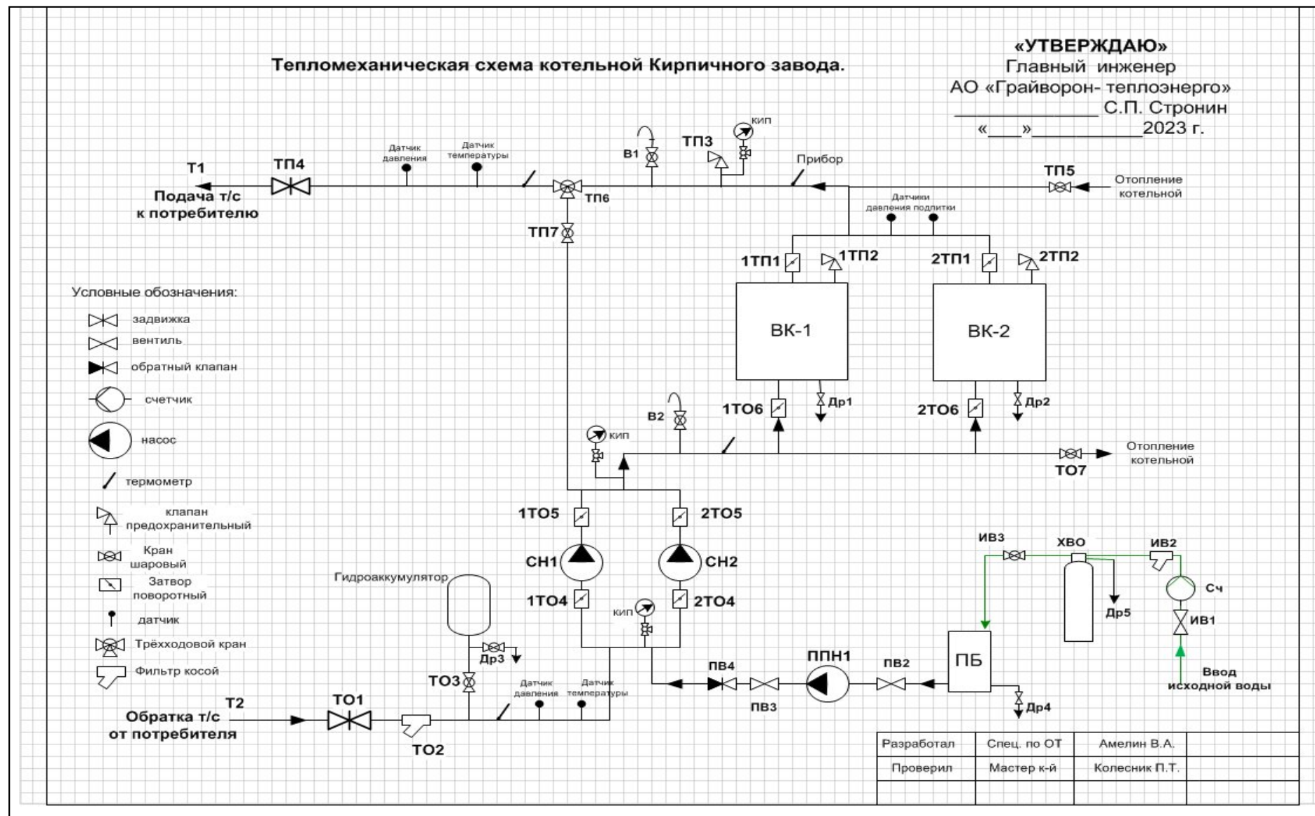
Рисунок 33. Тепловая схема котельной Кирпичный завод
