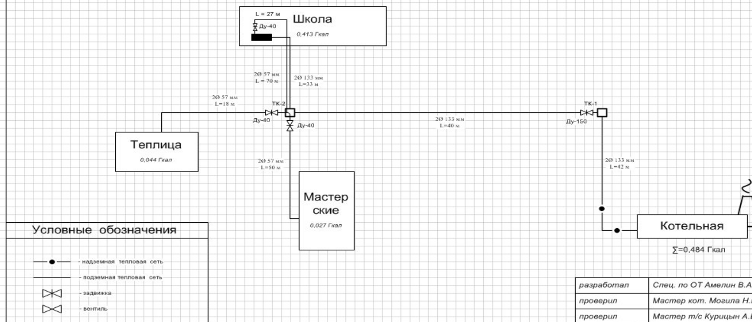
Рисунок 16. Зона действия котельной ТКУ с. Головчино (школа)
