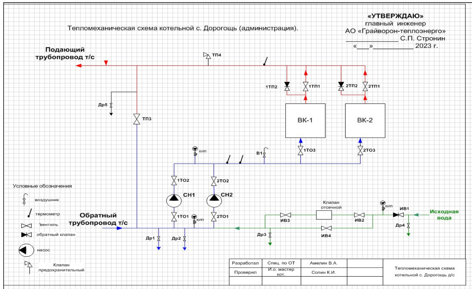
Рисунок 38. Тепловая схема котельной с. Дорогощ (администрация)
