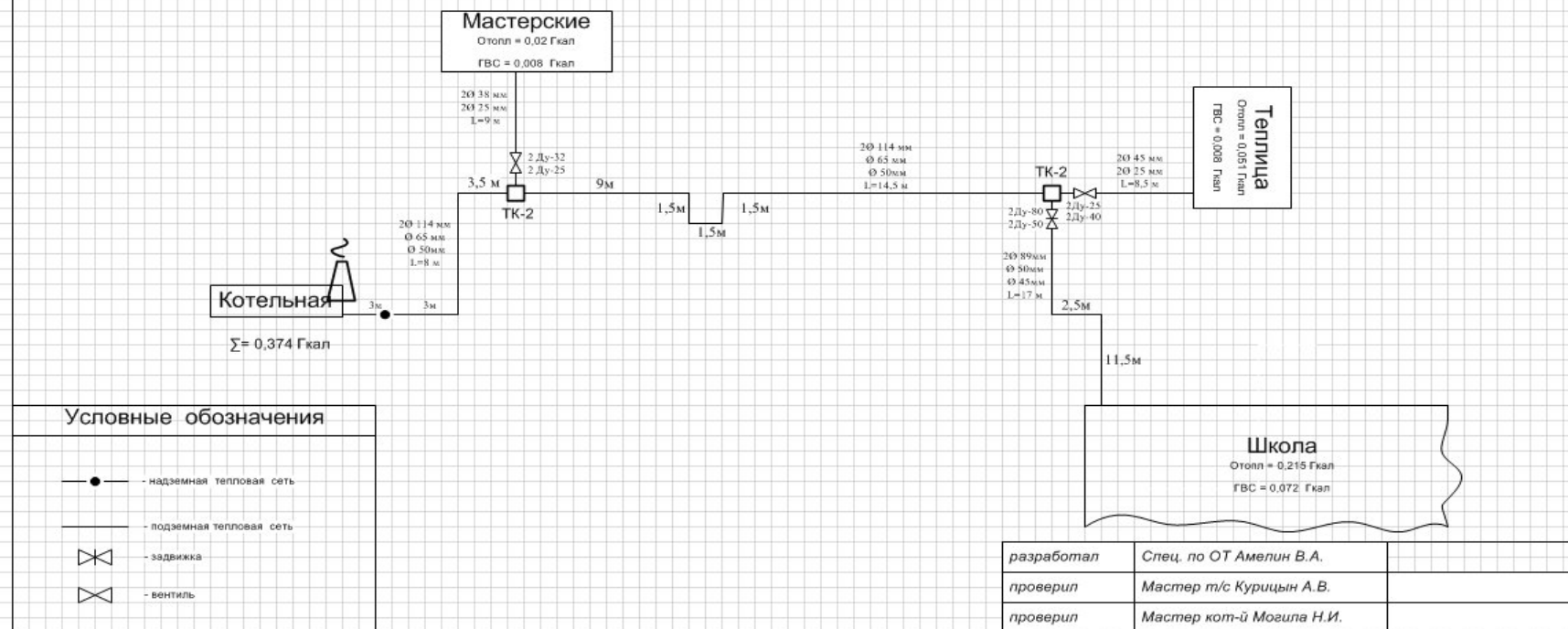
Рисунок 20. Зона действия котельной с. Доброе (школа)
