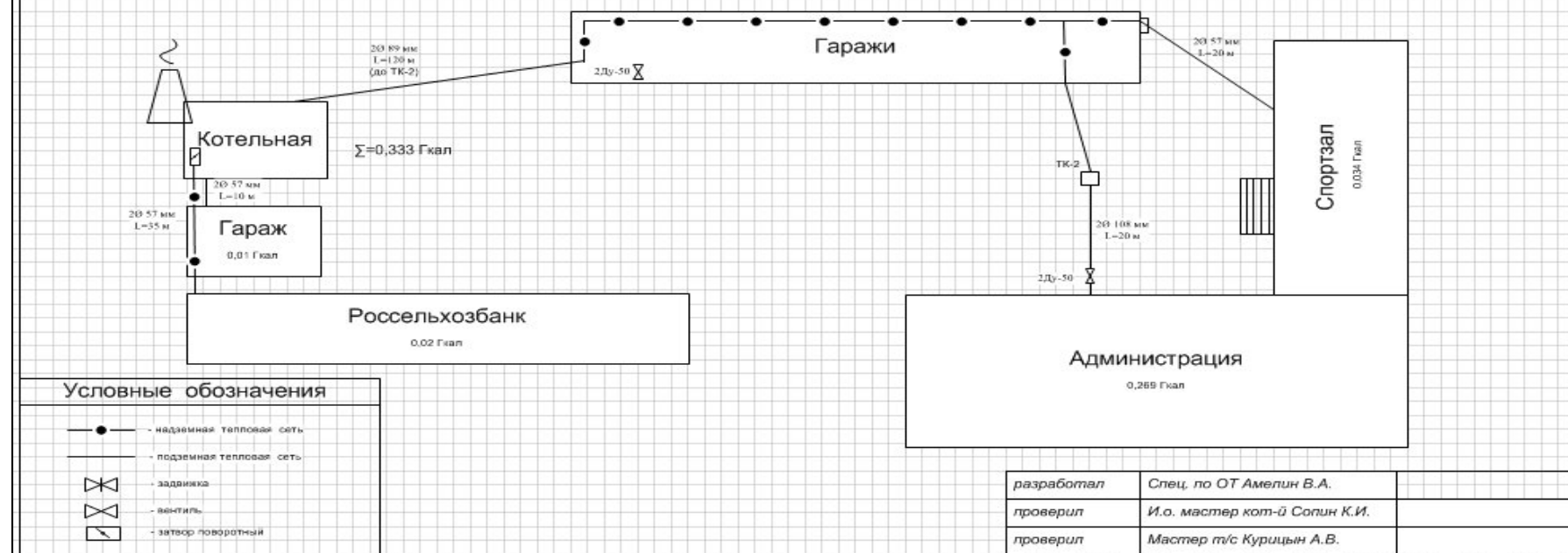
Рисунок 5. Зона действия котельной администрации округа
