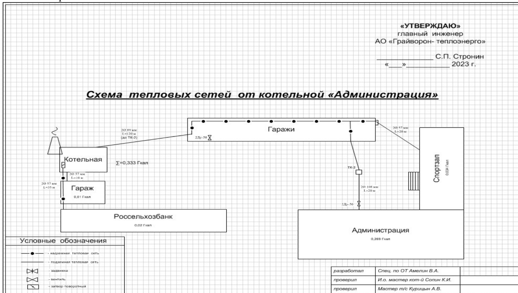
Рисунок 47. Схема тепловых сетей котельной Администрация муниципального округа
