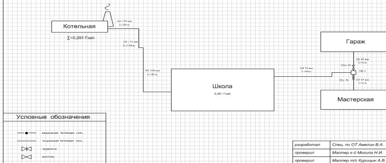
Рисунок 17. Зона действия котельной пос. Горьковский
