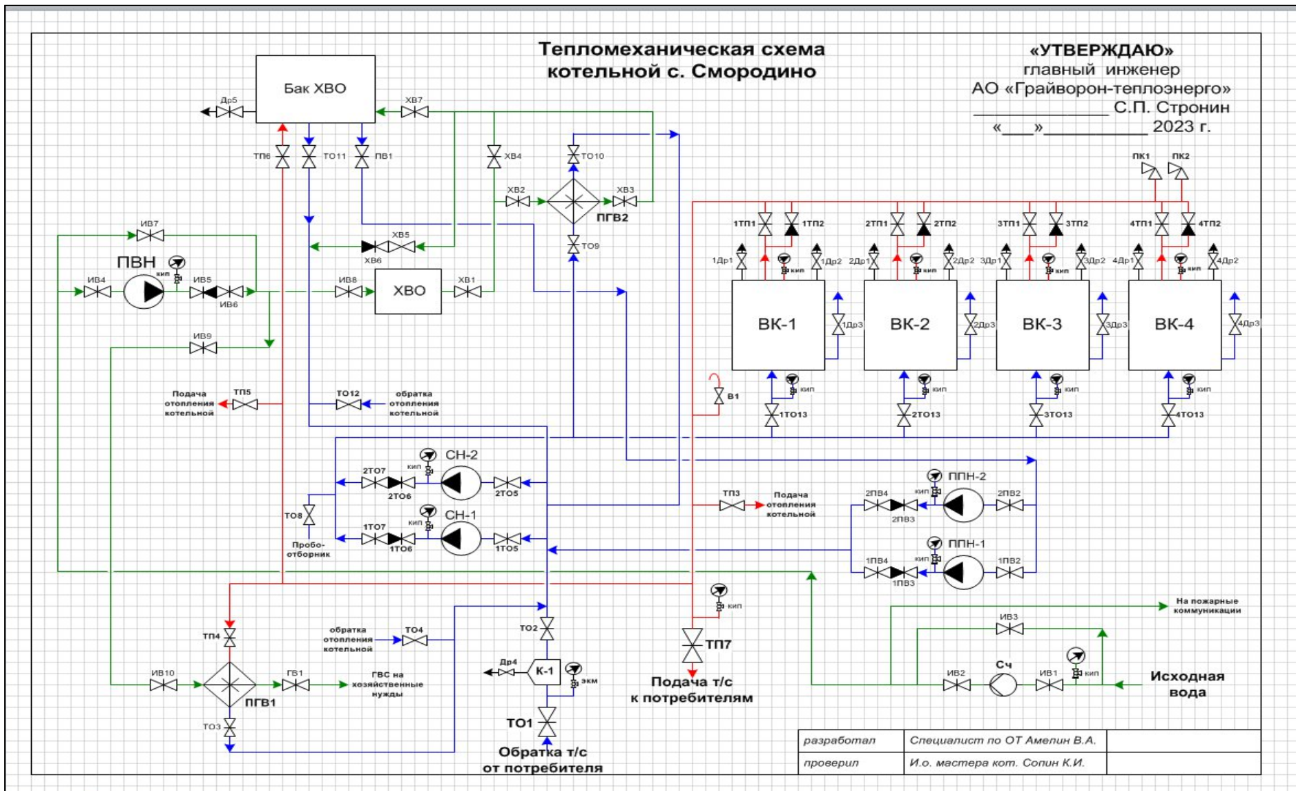
Рисунок 41. Тепловая схема котельной с. Смородино
