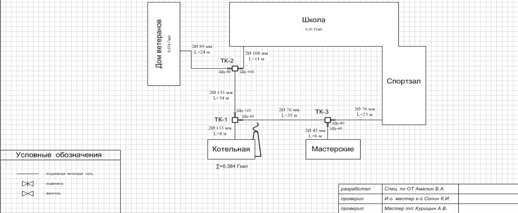
Рисунок 13. Зона действия котельной с. Мокрая Орловка
