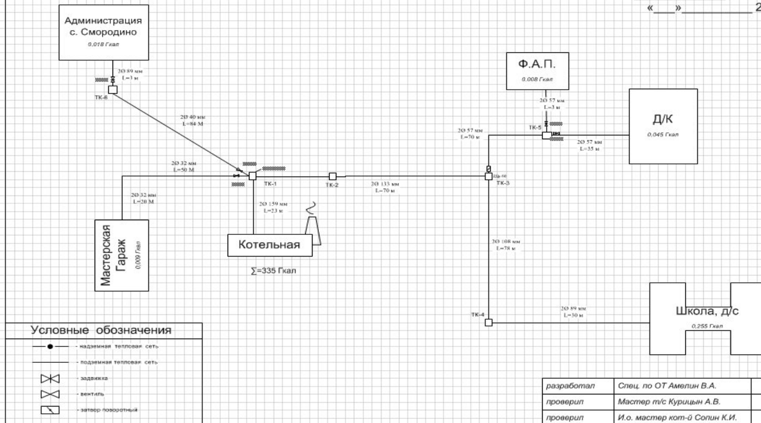
Рисунок 12. Зона действия котельной с. Смородино
