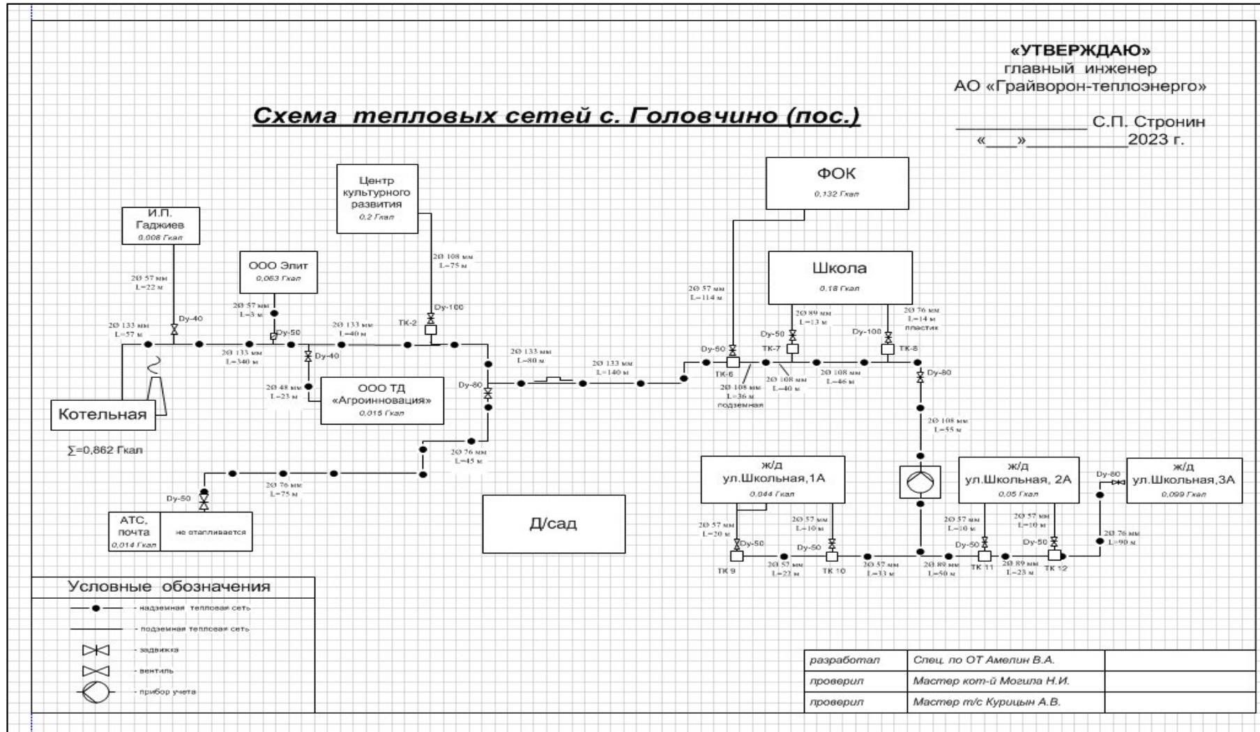
Рисунок 56. Схема тепловых сетей котельной с. Головчино (поселок)
