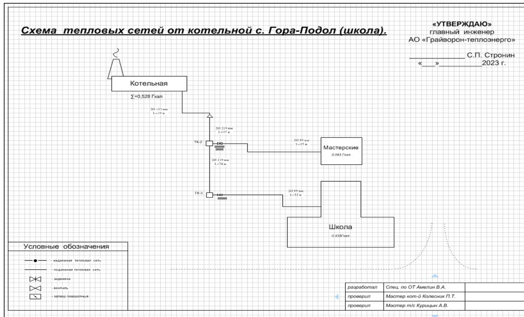
Рисунок 50. Схема тепловых сетей котельной с. Гора-Подол (школа)
