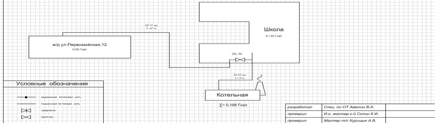
Рисунок 18. Зона действия котельной с. Дорогощь (школа)
