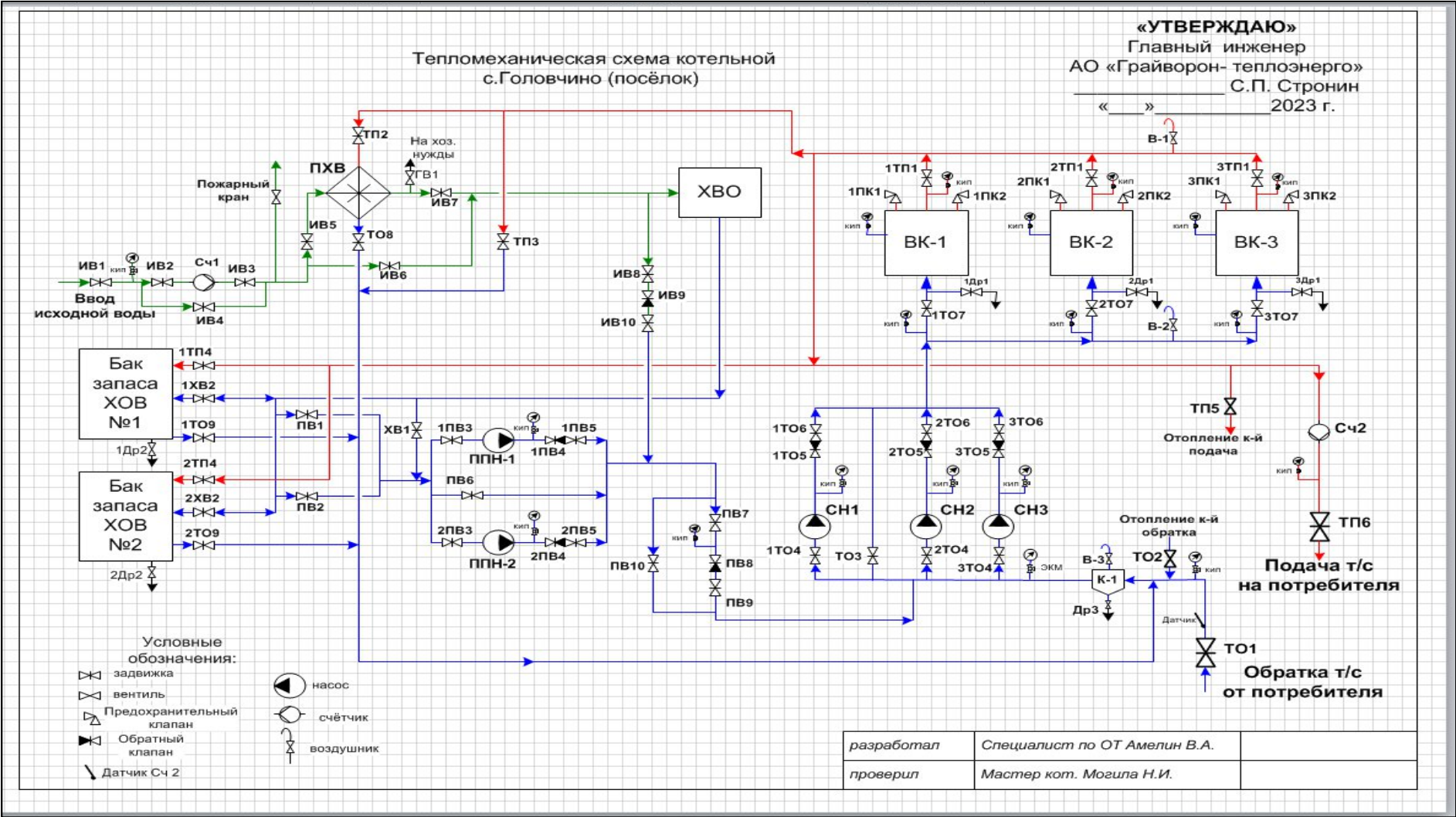
Рисунок 25. Тепловая схема котельной Головчино (поселок)
