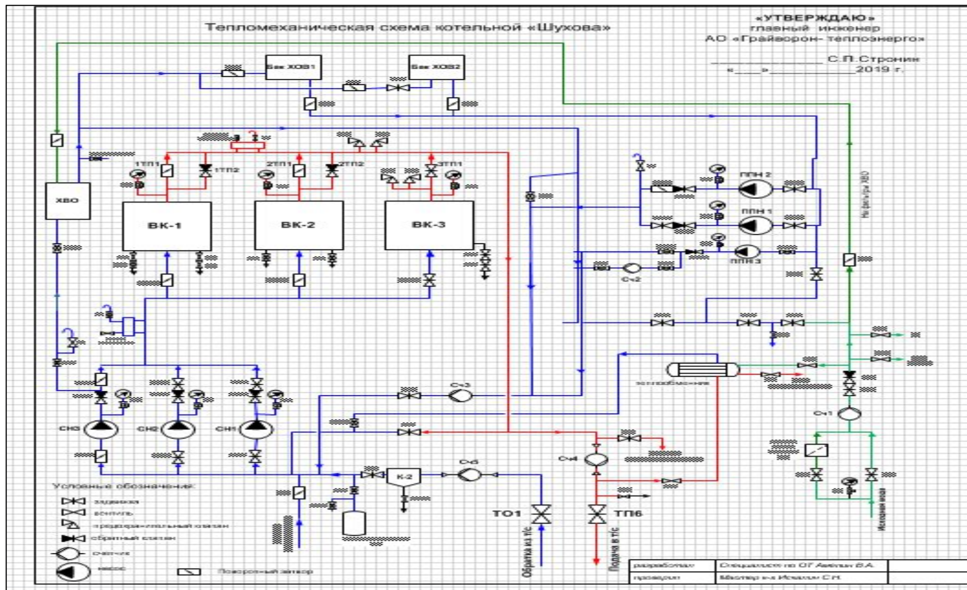
Рисунок 42. Тепловая схема котельной «Шухова»
