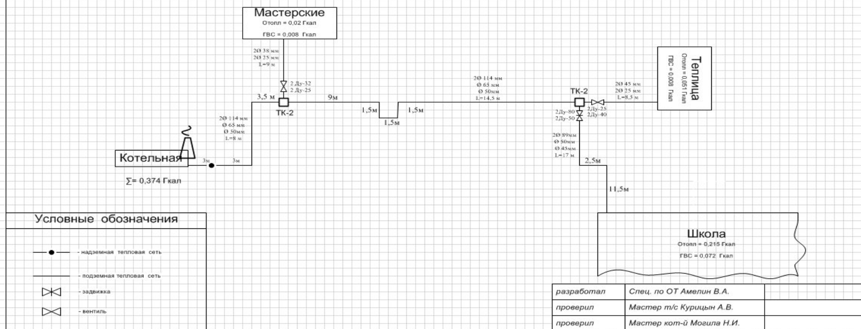
Рисунок 20. Зона действия котельной с. Доброе (школа)
