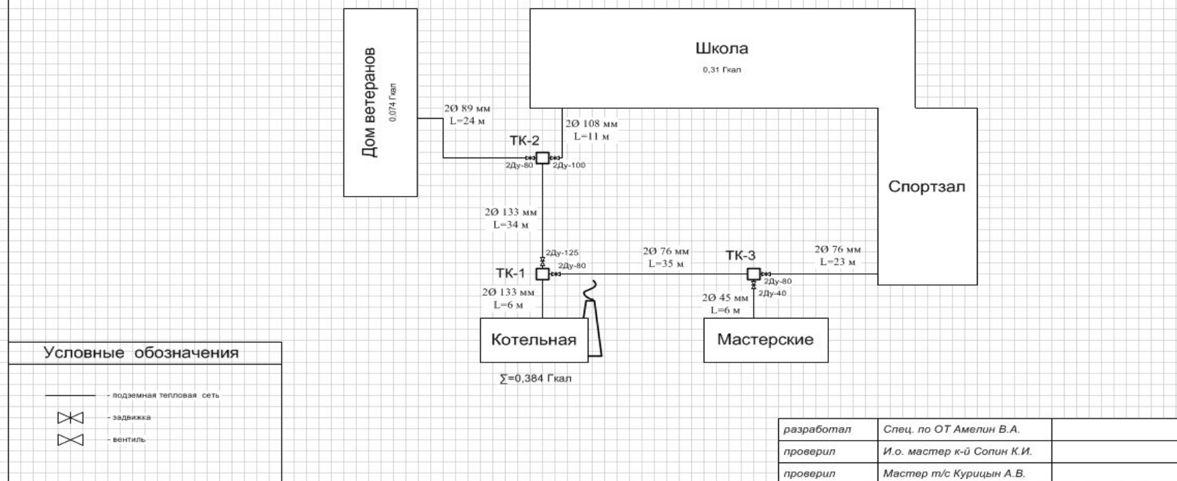
Рисунок 13. Зона действия котельной с. Мокрая Орловка
