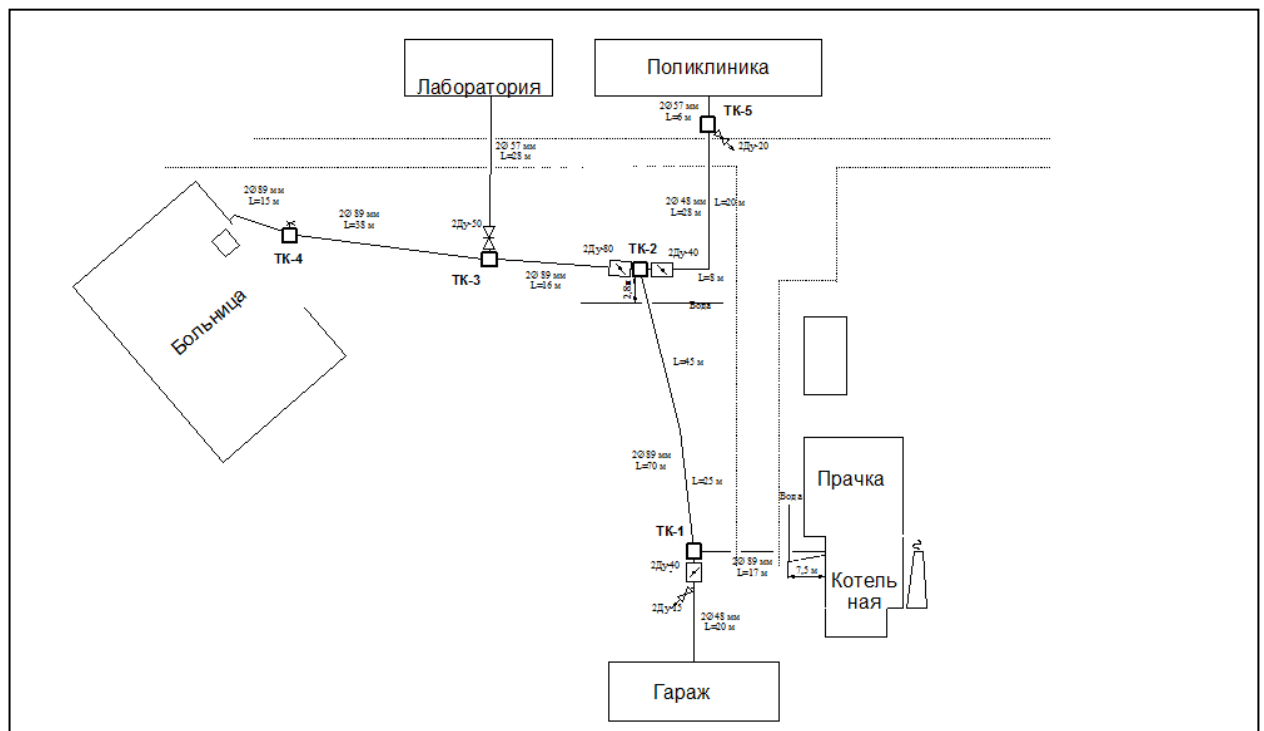
Рисунок 14. Зона действия котельной с. Головчино (больница)
