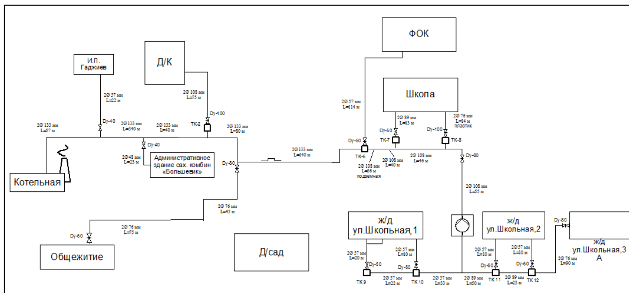
Рисунок 12. Зона действия котельной с. Мокрая Орловка
