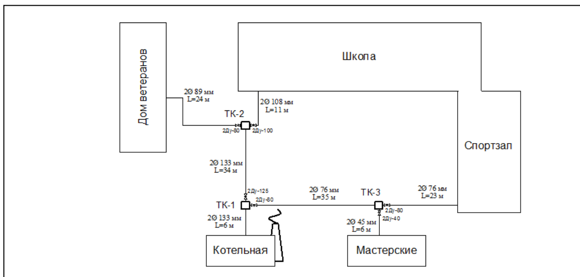
Рисунок 12. Зона действия котельной с. Мокрая Орловка
