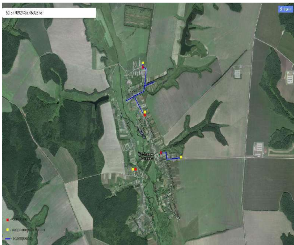
Рисунок 20. Схема водоснабжения с. Почаево
