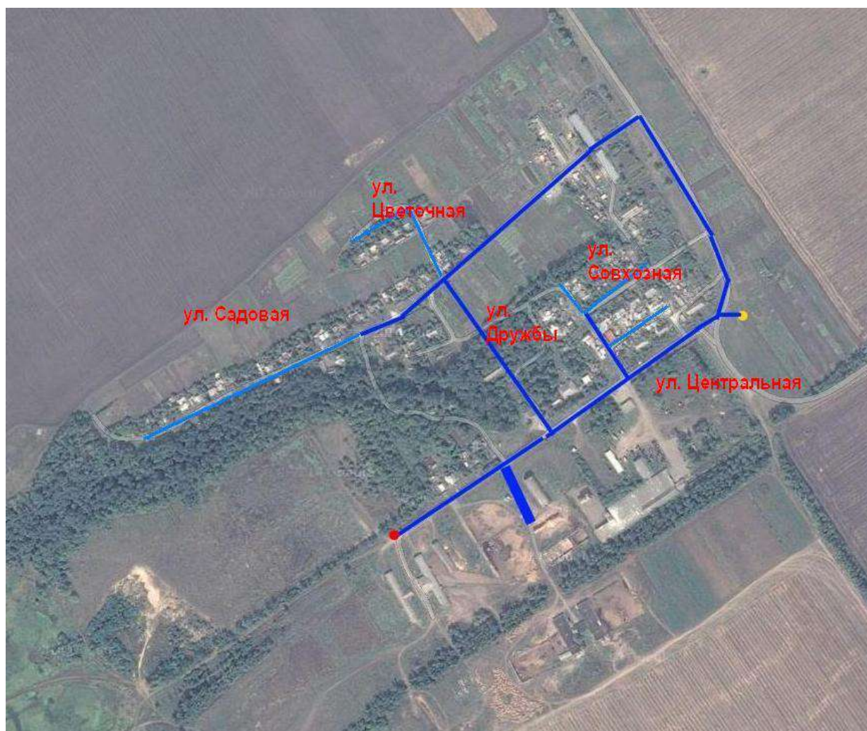
Рисунок 9. Схема водоснабжения п. Чапаевский
