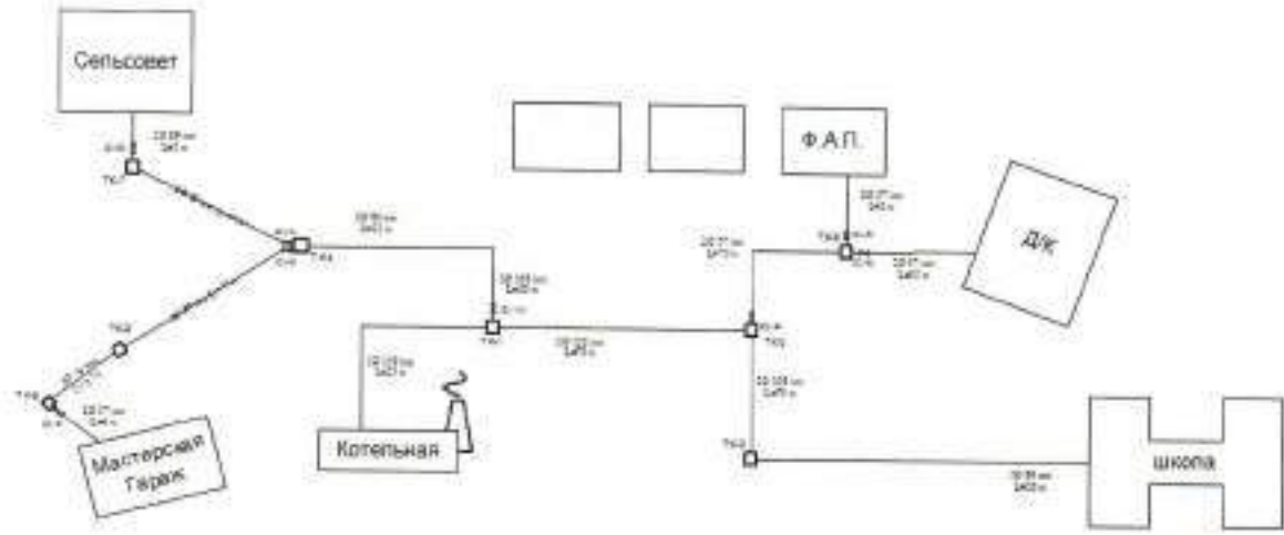
Рисунок 12. Зона действия котельной с. Смородино
