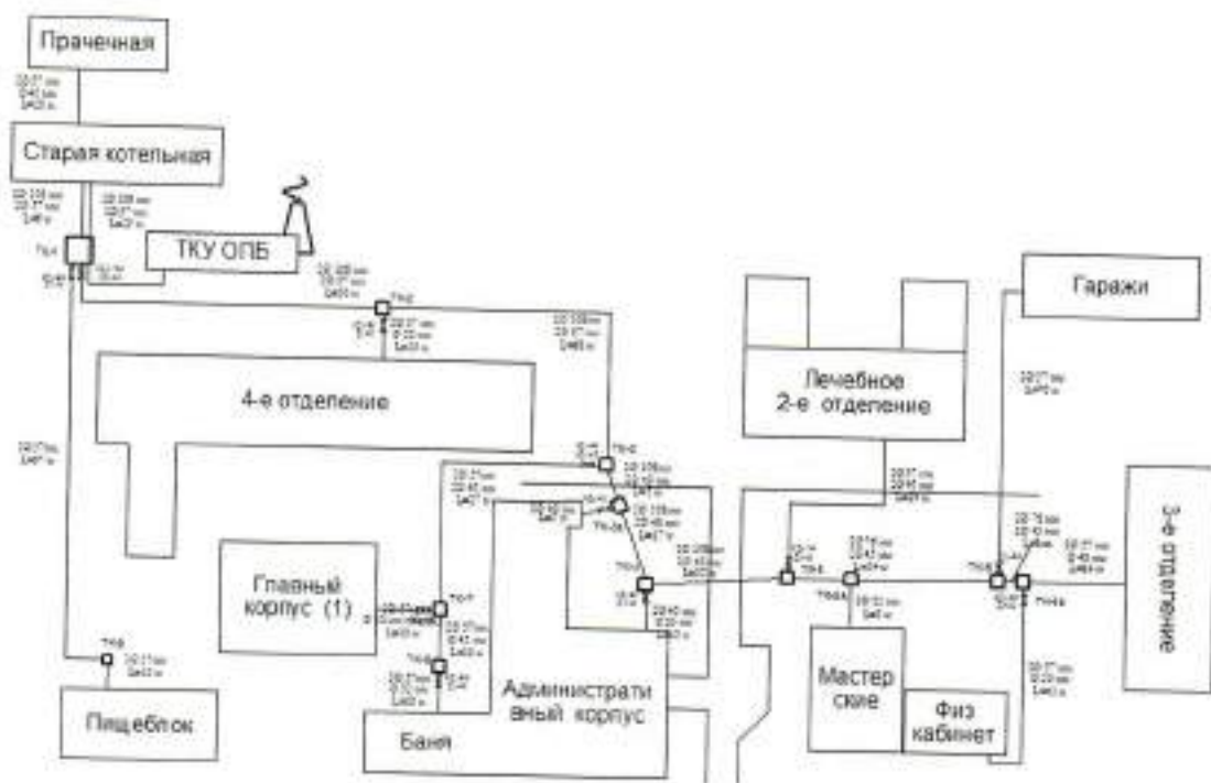
Рисунок 6. Зона действия котельной ОПБ ТКУ
