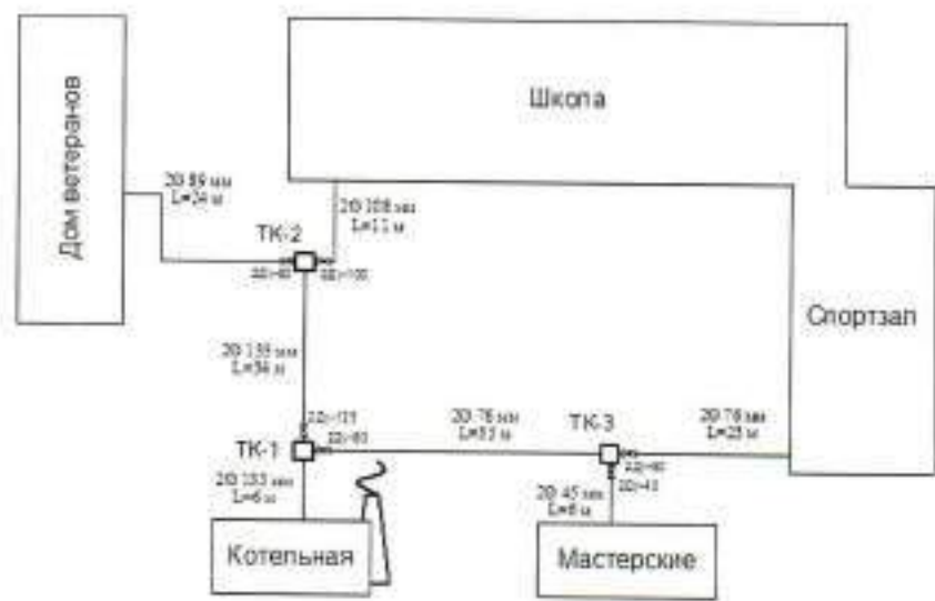
Рисунок 13. Зона действия котельной с. Мокрая Орловка
