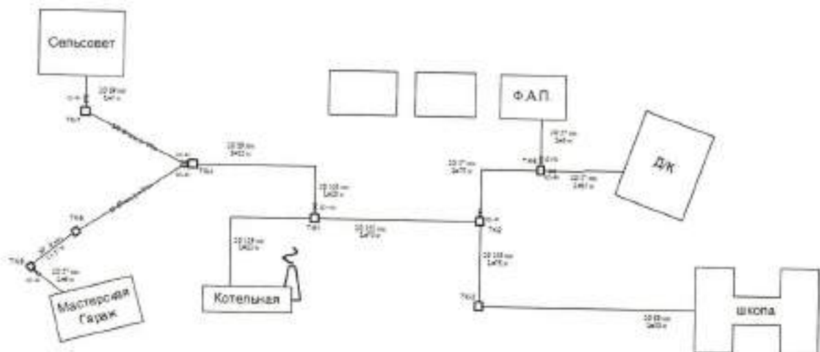
Рисунок 12. Зона действия котельной с. Смородино
