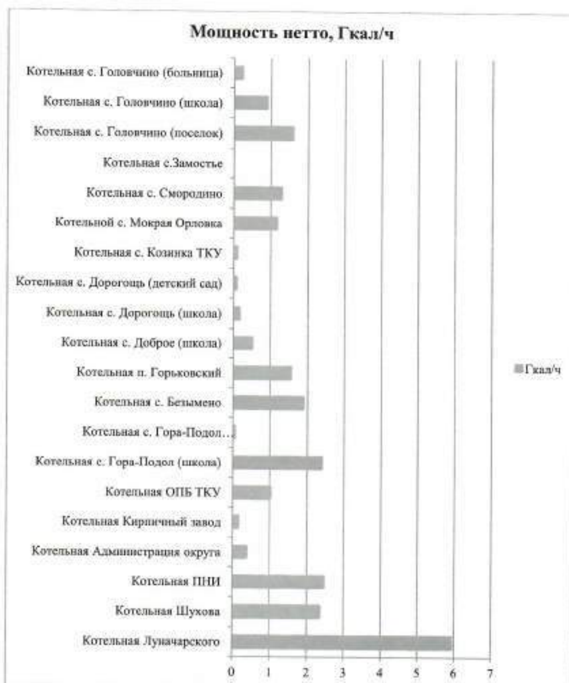
Рисунок 23 Мощность нетто котельных Грайворонского городского округа
