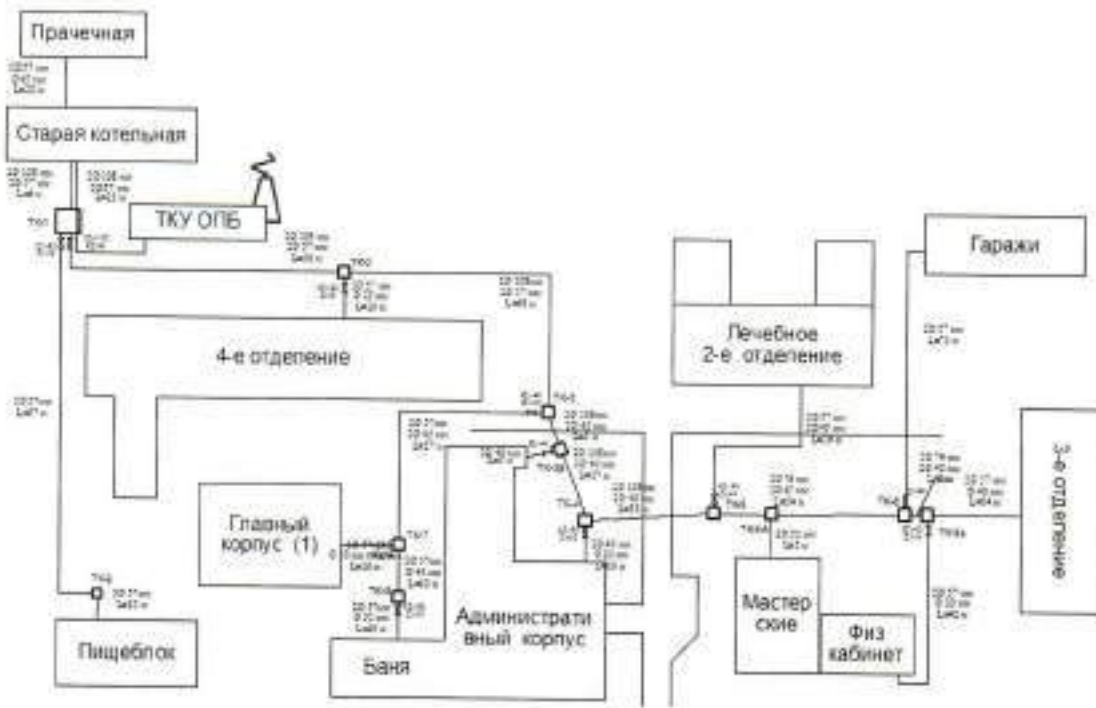
Рисунок 6. Зона действия котельной ОПБ ТКУ
