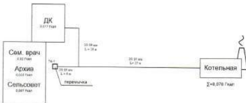
Рисунок 21. Зона действия котельной с. Замостье
