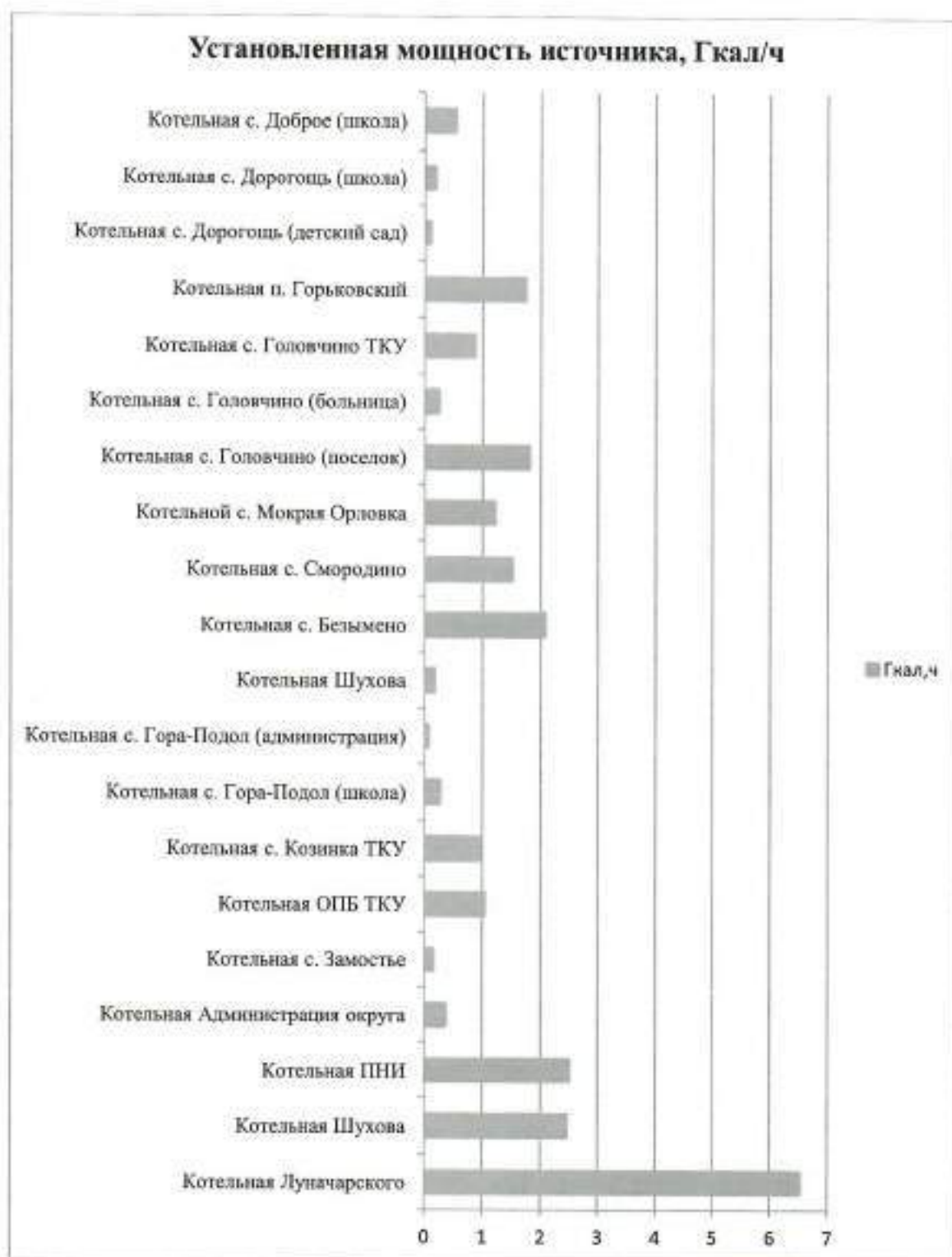
Рисунок 22 Установленная мощность котельных Грайворонского городского округа
