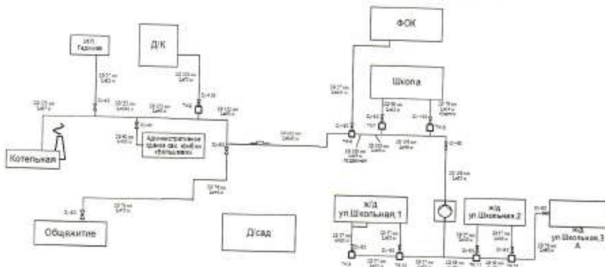
Рисунок 14. Зона действия котельной с. Головчино (поселок)
