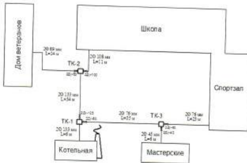
Рисунок 13. Зона действия котельной с. Мокрая Орловка
